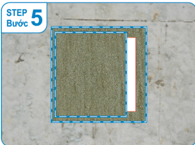
APPLY 2 COATS OF SMARTFLEX ONTO THE POLYESTER MAT. Quét 2 lớp SMARTFLEX bao phủ hết bề mặt toàn bộ lớp lưới gia cố
