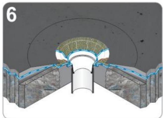
Protection mortar Cán vữa bảo vệ
