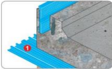
External Construction joint PVC Waterstop Băng cản nước PVC mặt ngoài mạch ngừng
