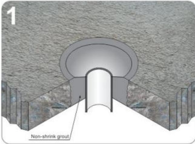
Down pipe treatment Ống thoát nước xuyên sàn
