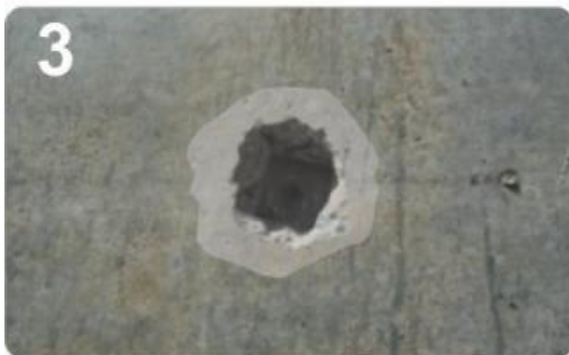
3 Apply 1 coat of latex onto the coin hole Quét 1 lớp phụ gia latex lên bề mặt lỗ ty
