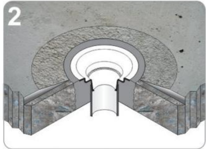
Sloping mortar 1.5 - 2.0% Cán vữa tạo dốc 1.5 - 2.0 %
