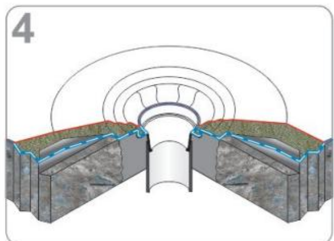
Polyester mat reinforcement for pipe Lưới polyester gia cố cổ ống
