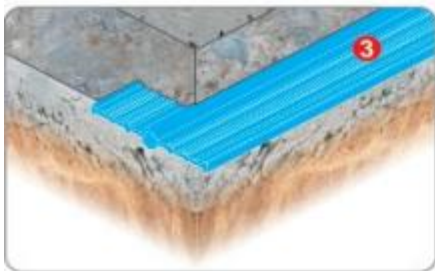
Internal Construction joint PVC Waterstop Băng cản nước PVC trung tâm mạch ngừng
